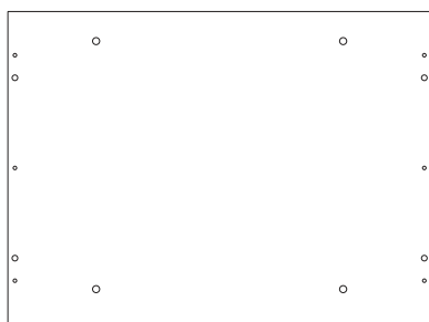
2 600 x 450 x 15 (1x)
